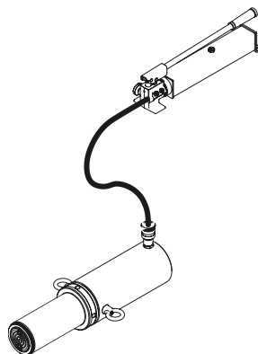
Figure 2 : Purger l'air du système
