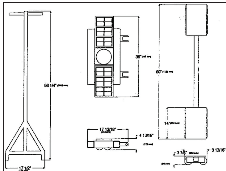
LP28–25 Ton Low Profile Dollie
