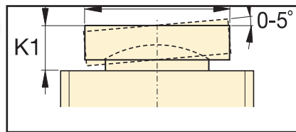
Optional Tilt Saddle
